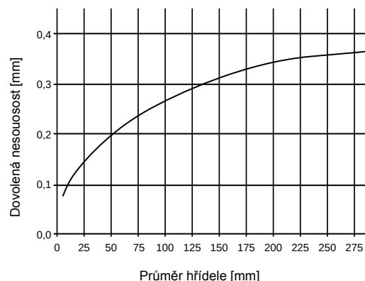
Statická výstřednost
