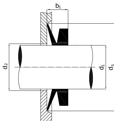
Rozměry V-kroužku
